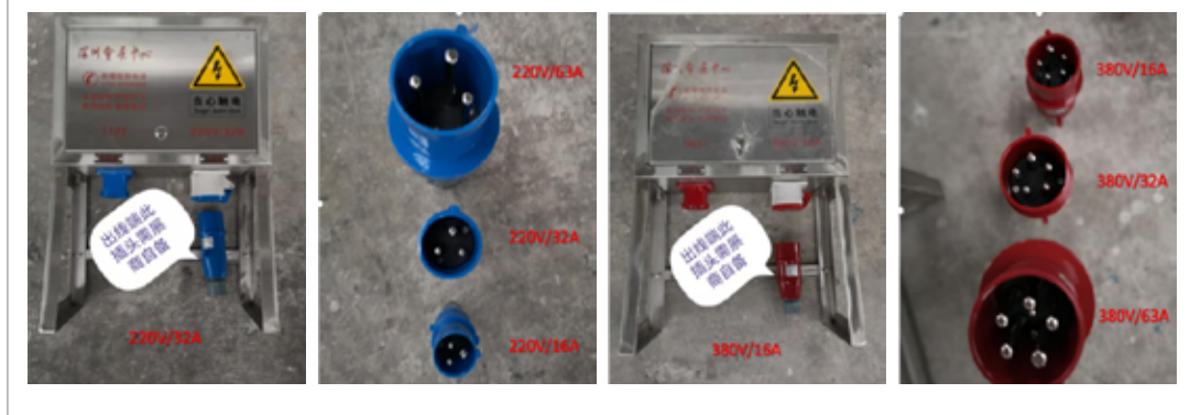
电力接驳示意图
